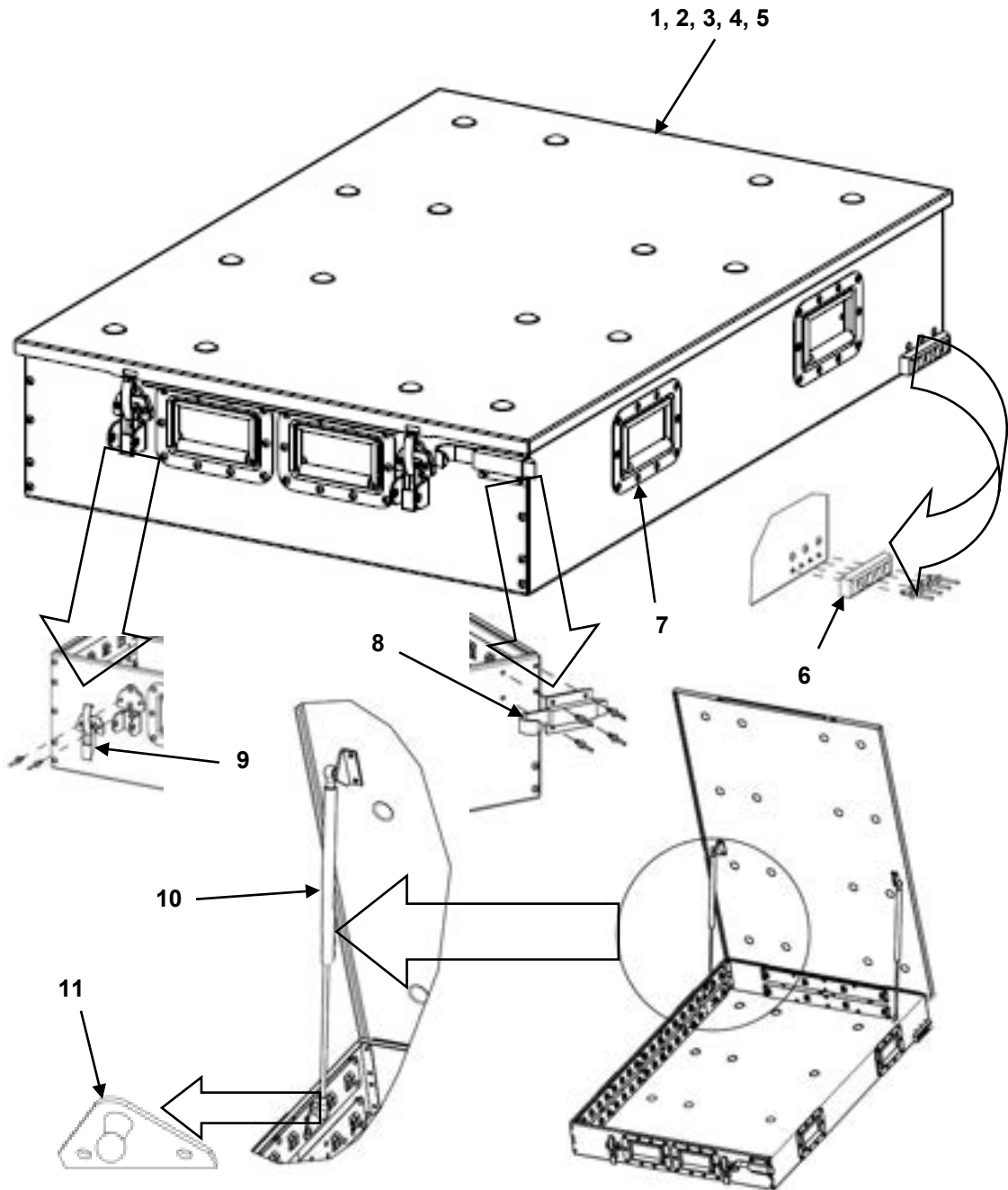
FIGURE 07 PDM 4", 6", 8", 12", 16" DRAWERS
