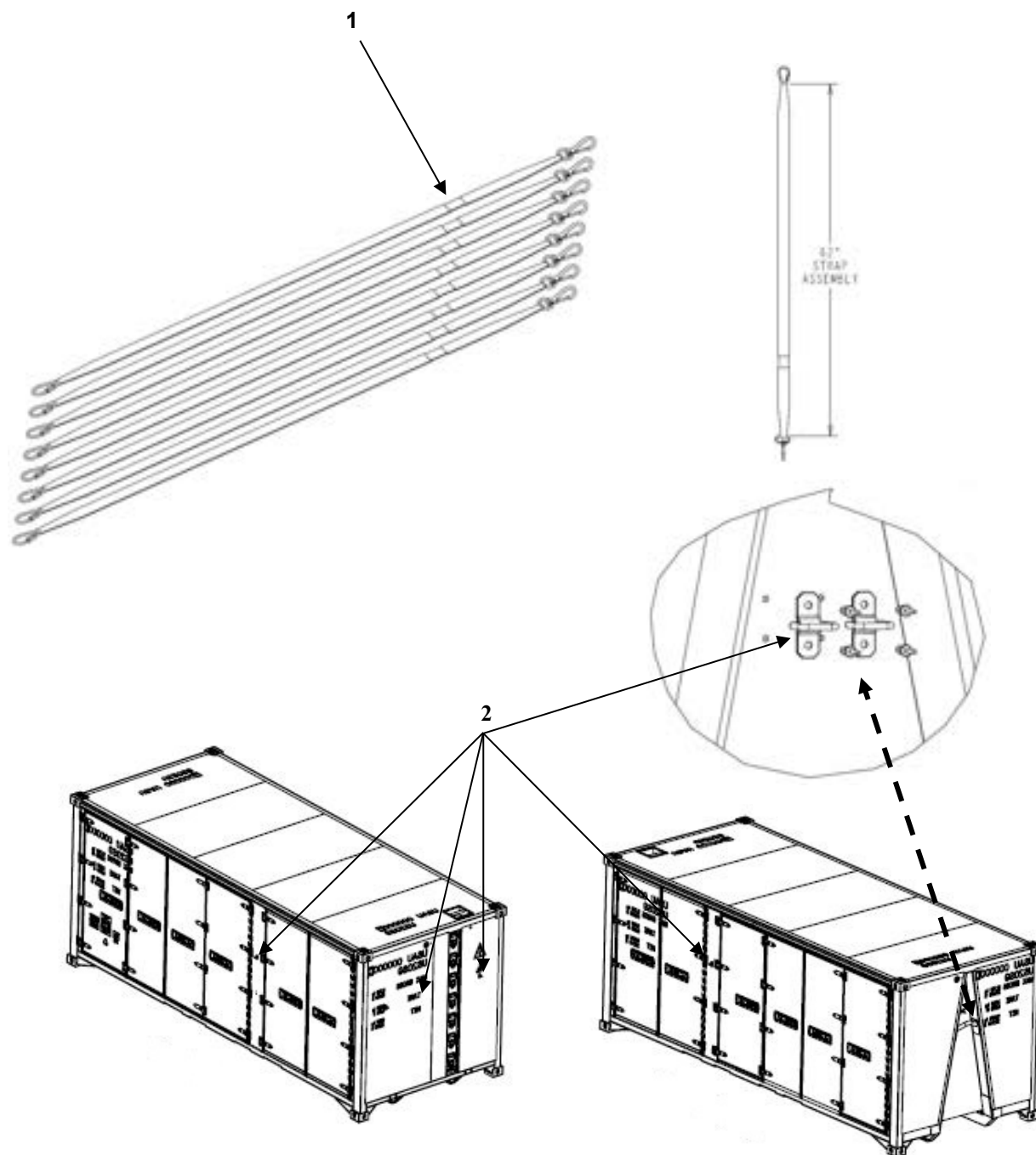
FIGURE 41 FPU 20-3 DOOR STRAPS
